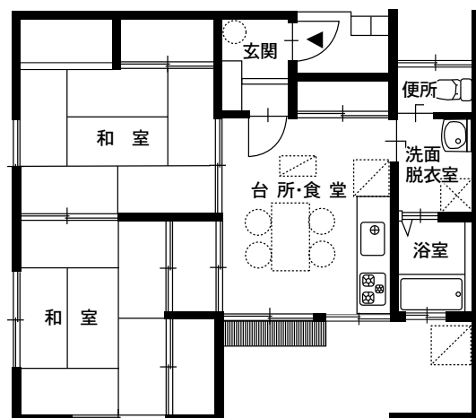
中村 2 D K (48.84㎡)
